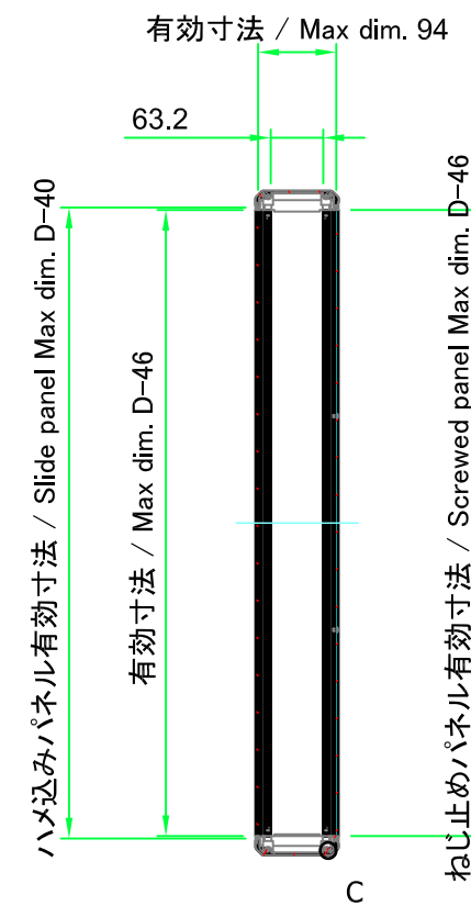
B-B ( 1 : 10 )
